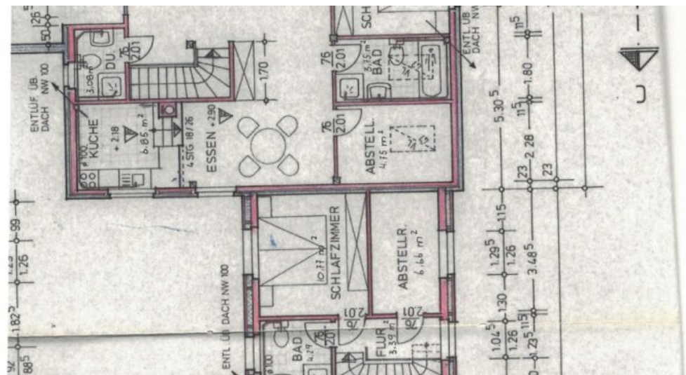
Grundriss oben
